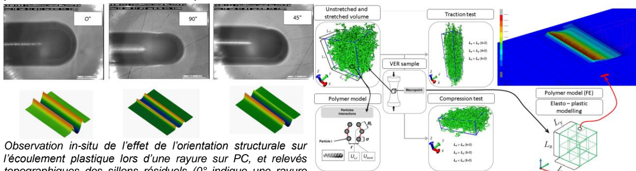
Estimation des propriétés volumiques à partir de simulation de dynamique moléculaire.
